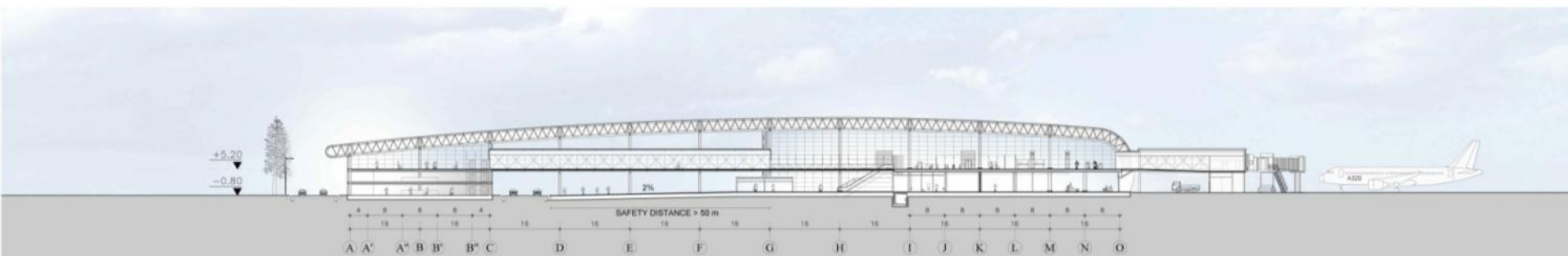
ПРОДОЛЬНЫЙ РАЗРЕЗ AA' LONGITUDINAL SECTION AA'
