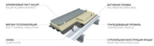
КОНСТРУКЦИЯ КРЫШИ ROOF STRUCTURE
